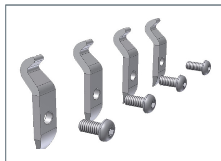
AM 425A K Greifhakensatz für 1 Radhalter, inkl. Schrauben
